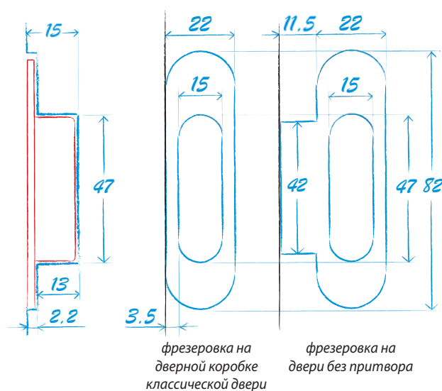
Взаимозаменяемость ответных планок Easy-matic на дверных коробках современных и классических дверей
