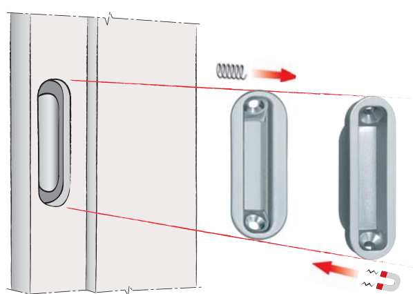
Взаимозаменяемость ответных планок Minimal на дверных коробках дверей с притвором
