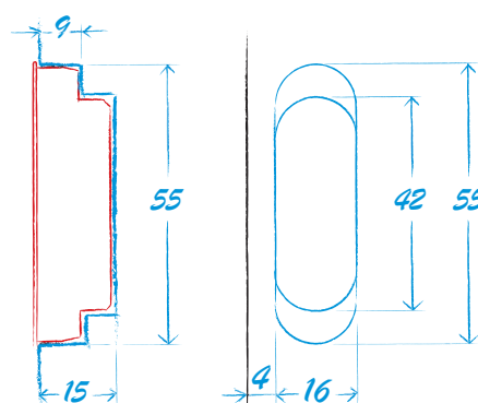
Пример фрезеровки на дверной коробке двери с притвором
